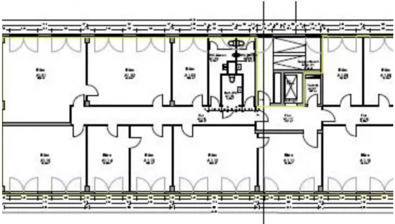
Grundrissplan 1.OG (Grundriss)
